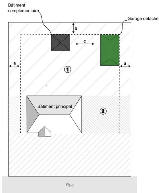
Croquis 5 : Garage détaché
