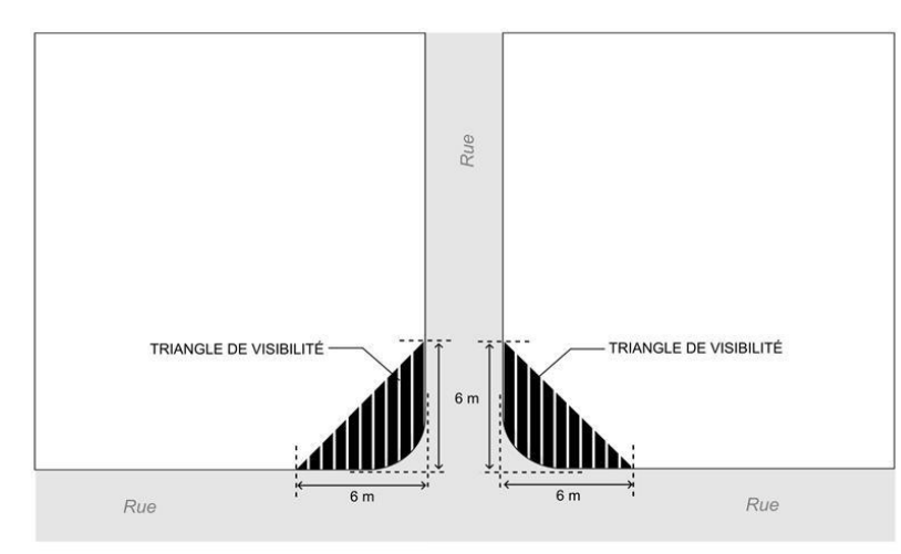
Croquis 11 : Triangle de visibilité
