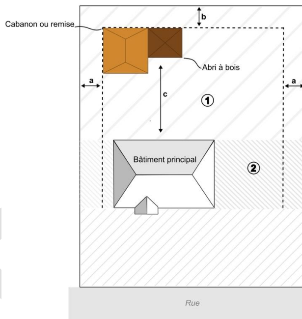
Croquis 1 : Abris à bois de chauffage
